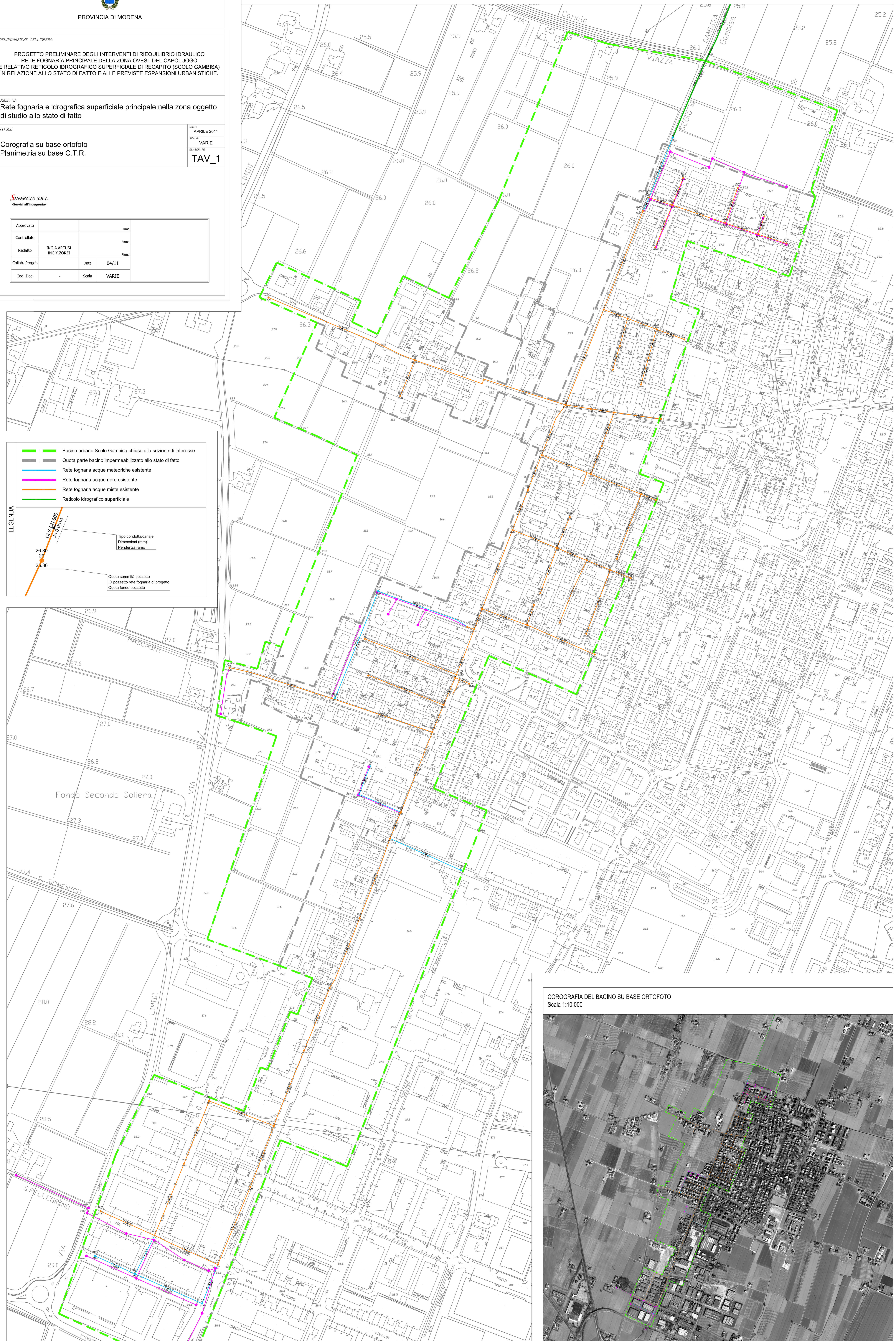
PLANIMETRIA RETE IDROGRAFICA E FOGNARIA PRINCIPALI ALLO STATO DI FATTO SU BASE C.T.R. Scala 1:2.000
