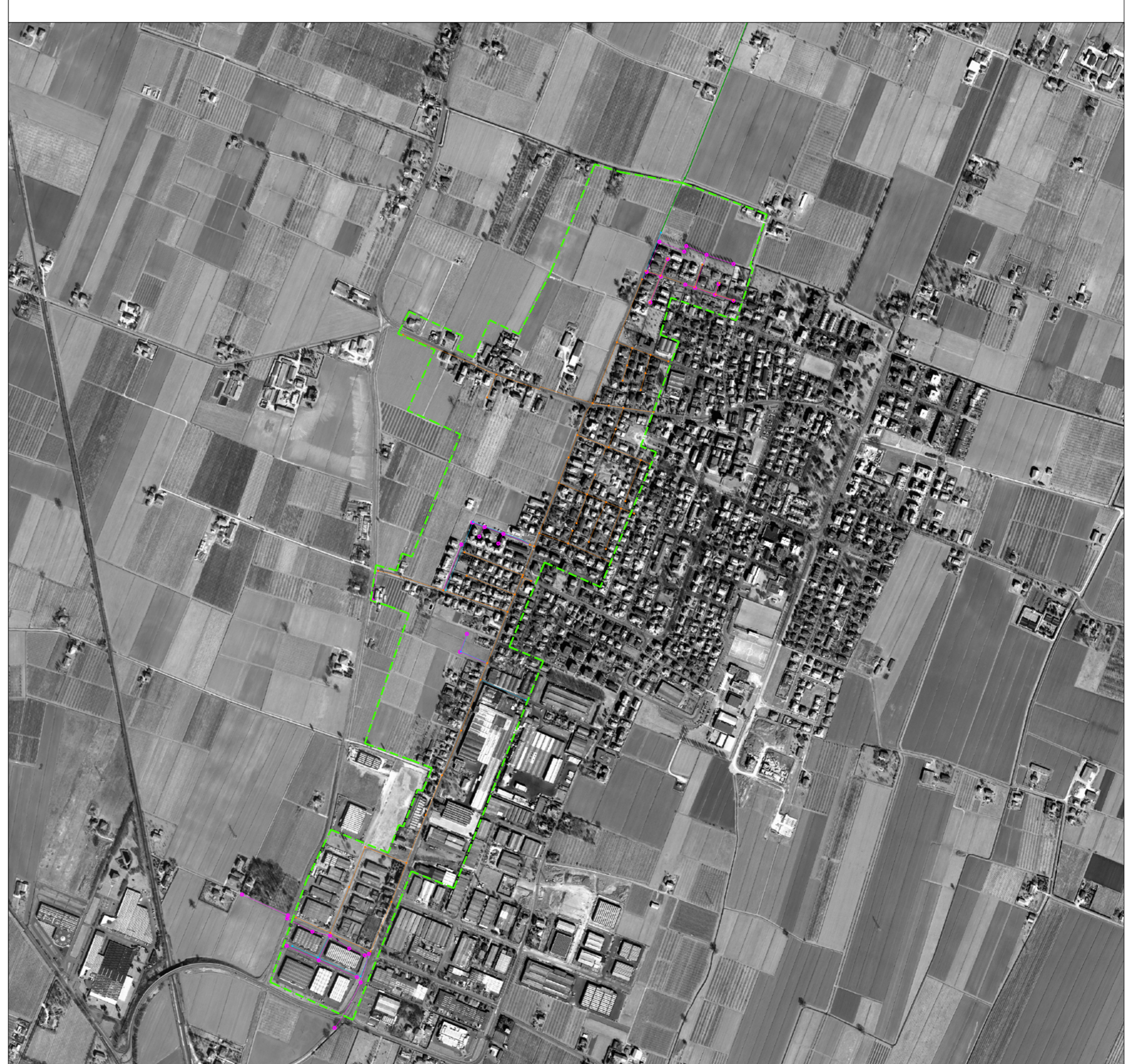
COROGRAFIA DEL BACINO SU BASE ORTOFOTO Scala 1:10.000
